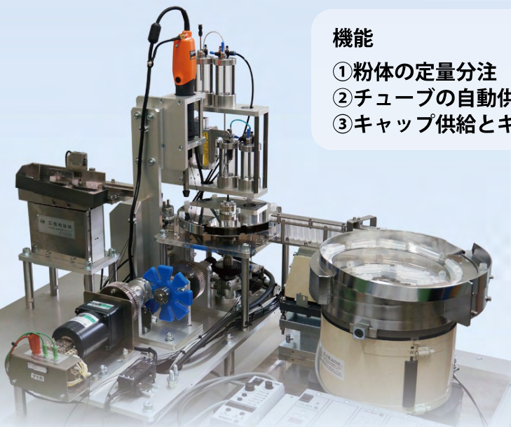
粉体定量分注ユニット
