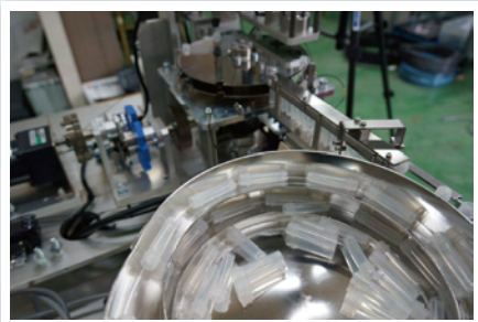
チューブ供給ユニット
