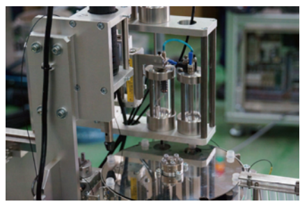
粉体定量分注ユニット
