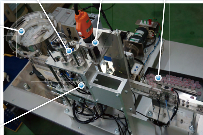
キャップ供給ユニット
